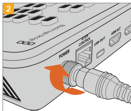
2 Sécurisez la connexion à l'ATEM Mini en serrant le connecteur à l'appareil.
