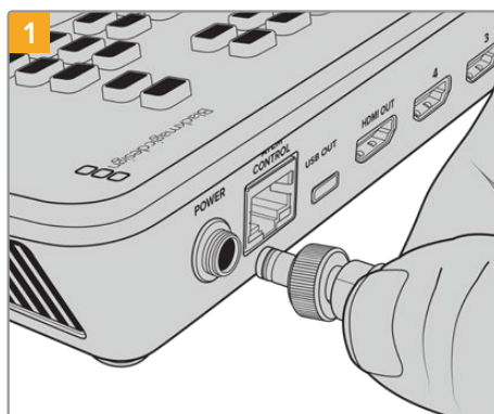
1 Connectez l'alimentation à l'entrée d'alimentation de l'ATEM Mini à l'aide du câble fourni.
