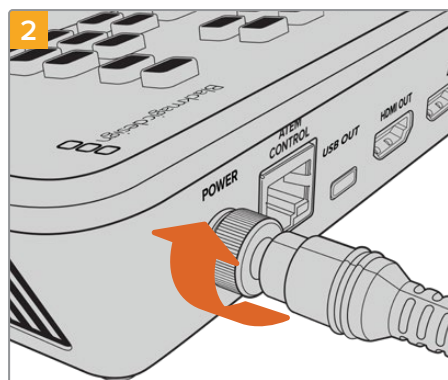
Enchufe el conector con firmeza.
