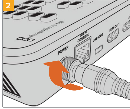
2 Konektör vidasını sıkıştırarak, konektörü ATEM Mini'ye sabitleyin.
